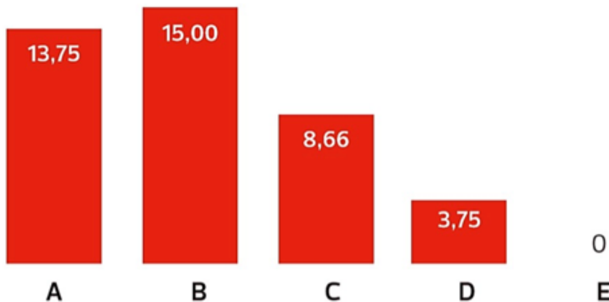
Figura 1 Distribuição da resistência média à compressão simples nas amostras testadas RESISTÊNCIA MÉDIA À COMPRESSÃO SIMPLES (kg/cm 2 )
